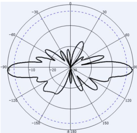
2400-2500MHz
